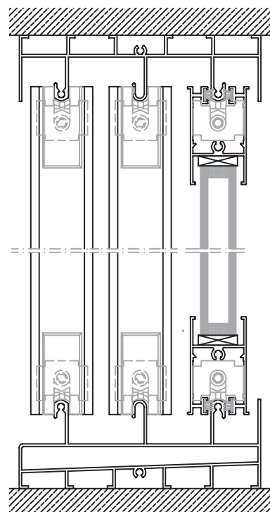
CORTE HORIZONTAL escala 1:3
