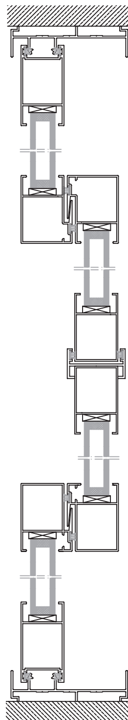
CORTE HORIZONTAL escala 1:3
