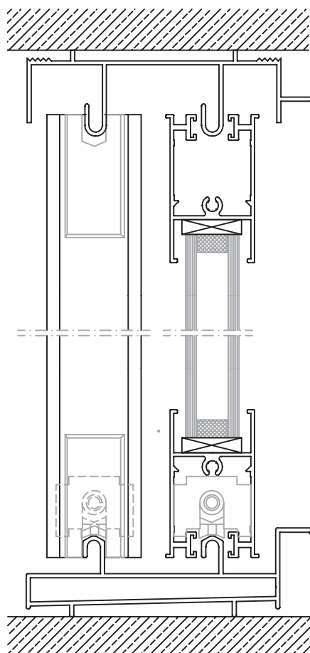
CORTE VERTICAL escala 1:2
