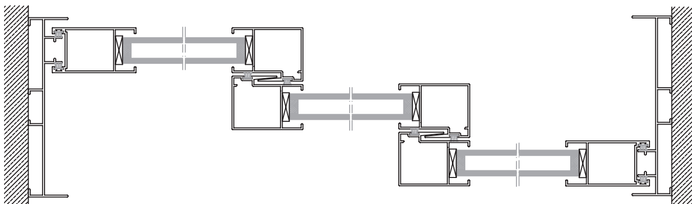
CORTE VERTICAL escala 1:3
