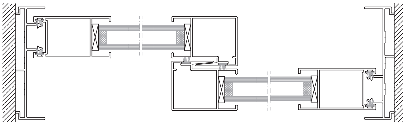
CORTE HORIZONTAL escala 1:2
