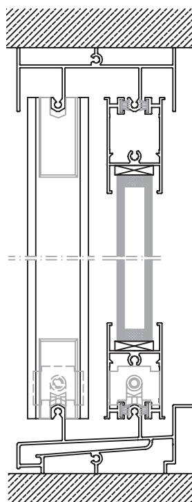
CORTE VERTICAL escala 1:3
