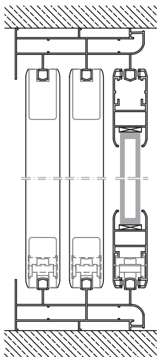
CORTE VERTICAL escala 1:3
