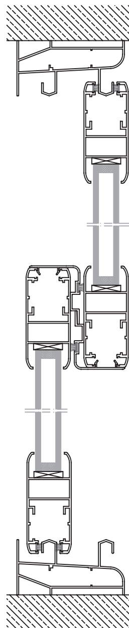
CORTE HORIZONTAL escala 1:3
