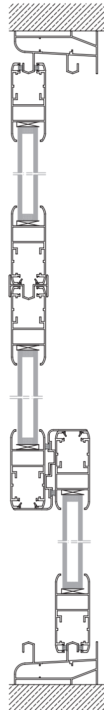
CORTE HORIZONTAL escala 1:4
