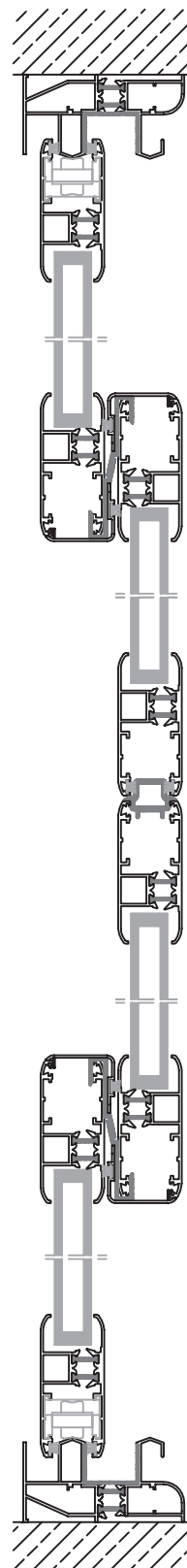
CORTE HORIZONTAL escala 1:4
