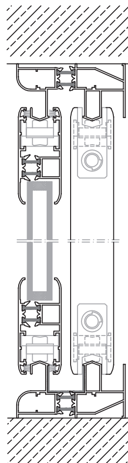
CORTE VERTICAL escala 1:3
