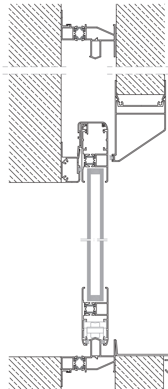
CORTE HORIZONTAL escala 1:3
