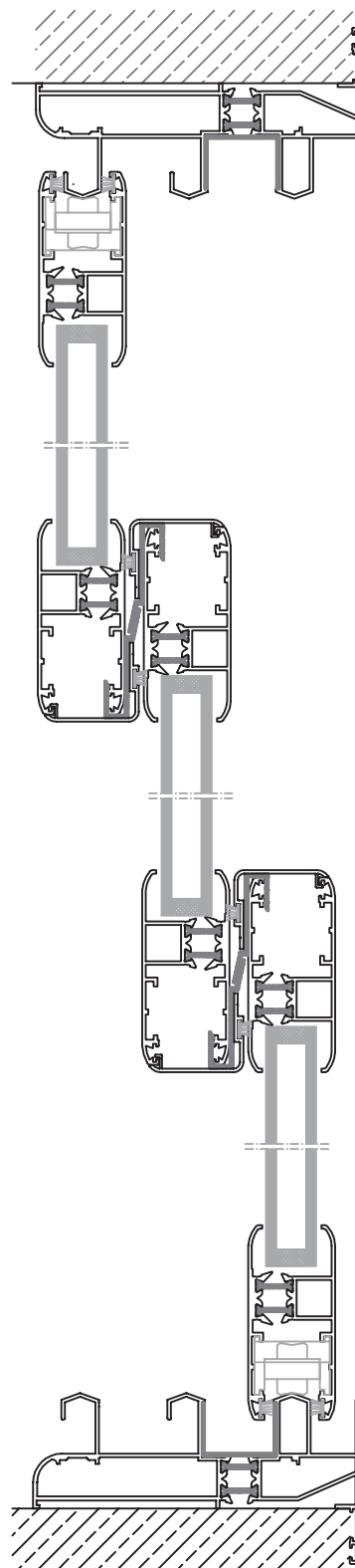
CORTE HORIZONTAL escala 1:3
