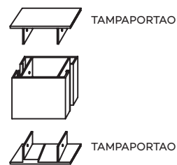
DETALHE B
